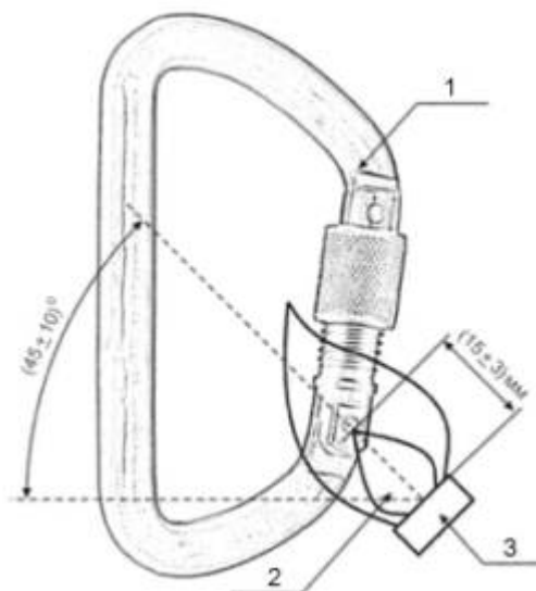
1 - карабин; 2 - голубой конус пламени; 3 - горелка Бунзена
