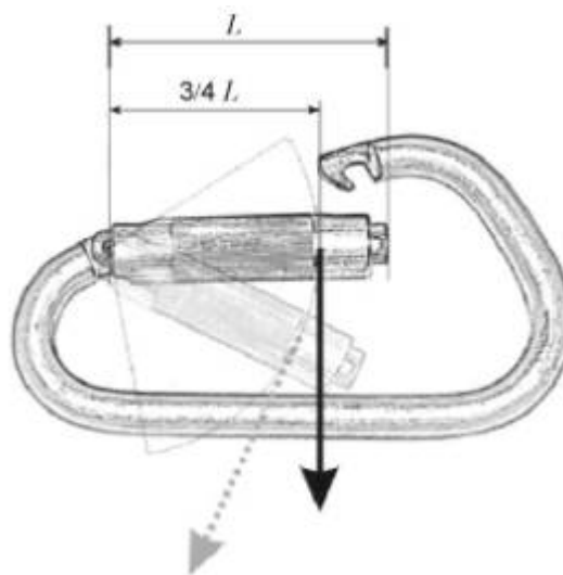
Рисунок 2 - Схема испытания усилия раскрытия затвора карабина
