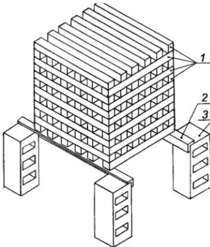
Рисунок Б.1 - Устройство деревянного штабеля (модельного очага) для проведения испытаний по тушению пожара класса А
