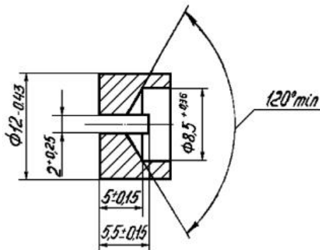
Рисунок А.1 - Насадок-распылитель
